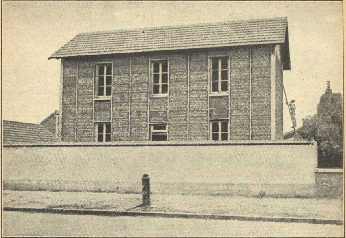
LA MAISON ISOTHERMIQUE EST COMPLÈTEMENT CLOSE ET COUVERTE Les murs attendent leur enduit ; mais telle qu'elle est, la construction est déjà suffisamment engageante.
