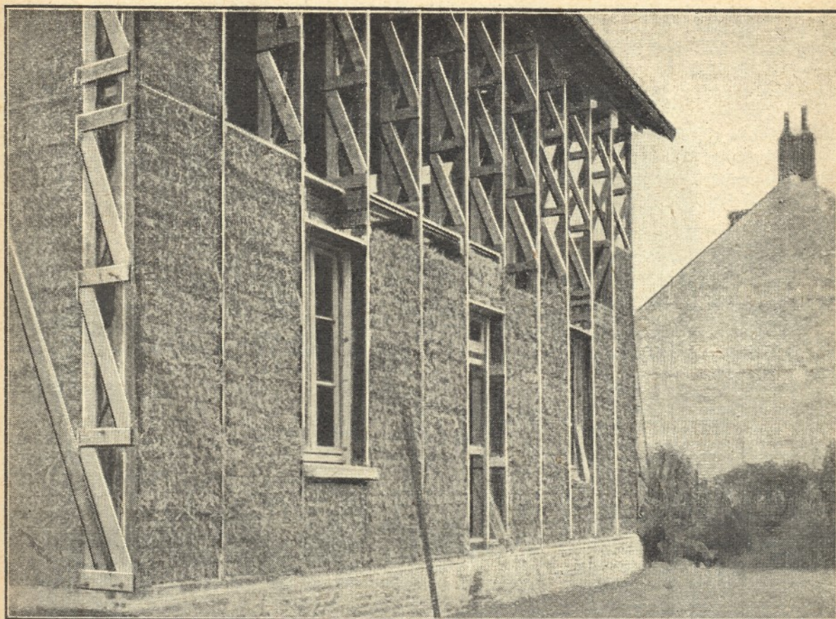
LES MURS DE LA MAISON ISOTHERMIQUE COMMENCENT A PRENDRE TOURNURE
